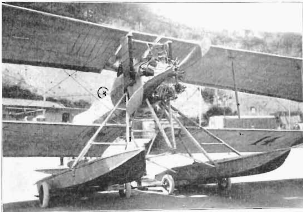
Ci-dessus : Breguet type H-U3 vu à Monaco en 1914. (Revue Aeronautics). Ci-dessous : « La Marseillaise » 1913. (Les Ailes).
