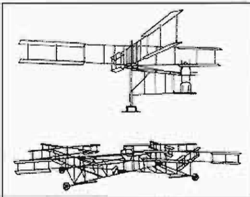
Le gyroplane Breguet-Richet n° 1 (1907). En bas vue générale, en haut vue d'un rotor. (Musée de l'Air).
