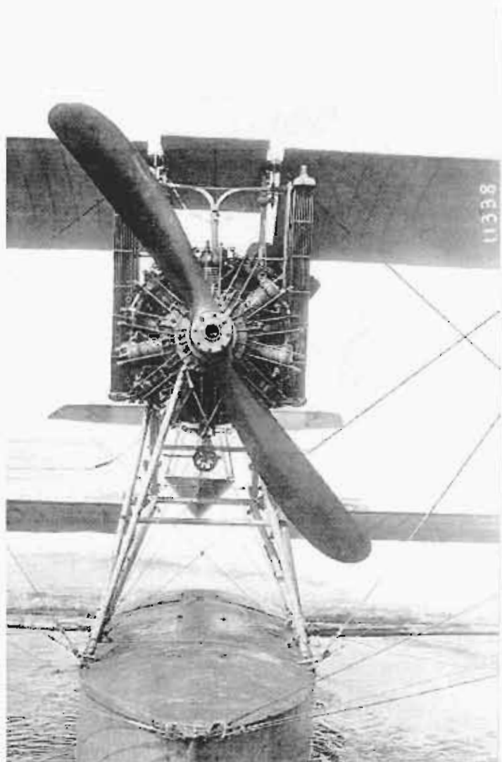
L'impressionnant moteur Salmson de 200 ch utilisé sur le Breguet H-U3 à Monaco et Deauville 1913. (Musée de l'Air).
