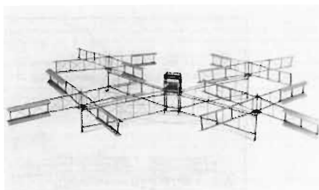
Plan du gyroplane Breguet-Richet n° 1. Le moteur est placé au centre. (Musée des Arts & Métiers).
