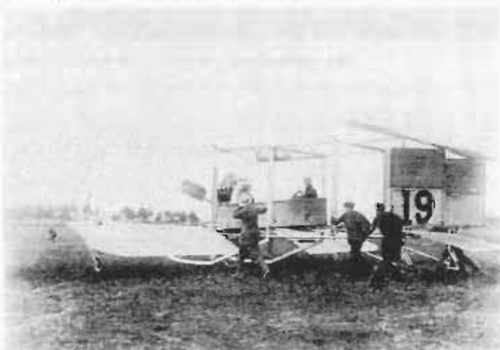
Le Breguet type I vu à Reims en 1909 possède un plan d'aile supérieure variable en incidence. (Musée de l'Air).
