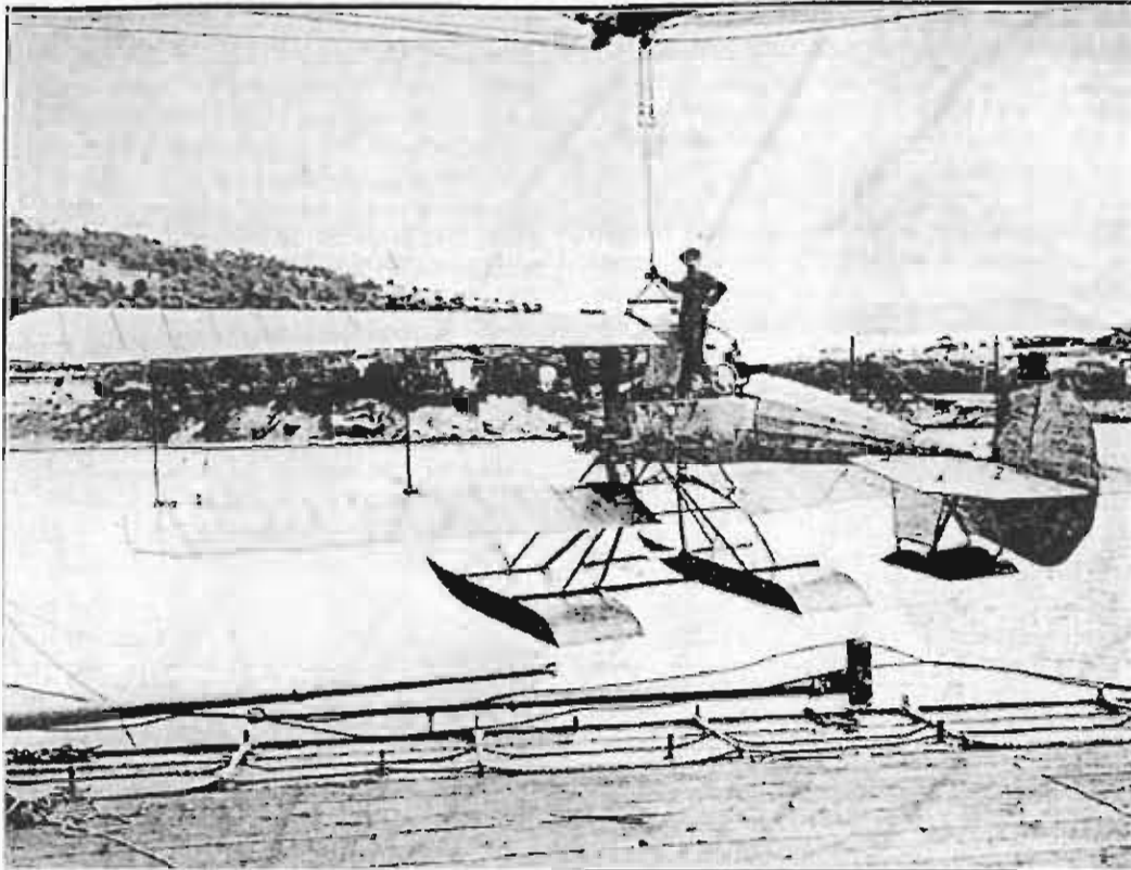
Vue arrière du H-U2 de Brégi à Monaco en avril 1913 lors de l'épreuve de halage. (L'Aérophile 1913).
