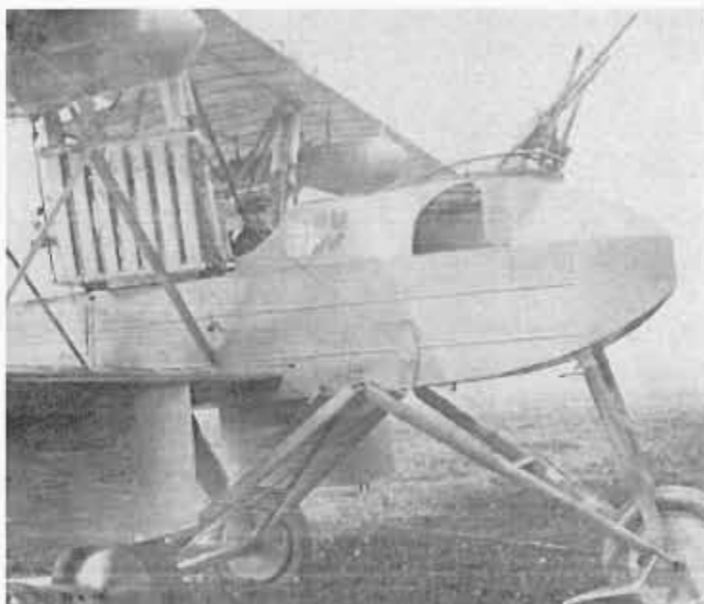
Le Breguet-Michelin type BUM à moteur Salmson de 130 ch. (Musée de l'Air).
