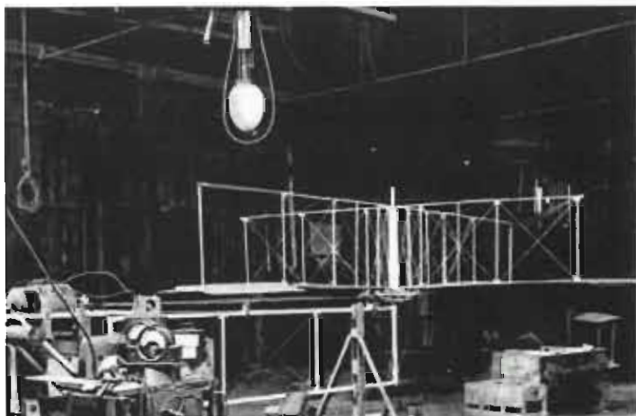
Balance aérodynamique construite par Louis Breguet en 1906 lui permettant d'étudier les profils d'aile. (Archives de l'Aéro-Club de France).
