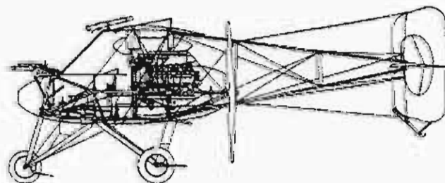
Le Breguet type 5, chasseur d'escorte à canon de 37 mm avant. (Manuel d'aviation de la première guerre mondiale).
