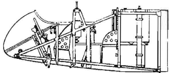
Nacelle du Breguet BUM de bombardement. (1916).
