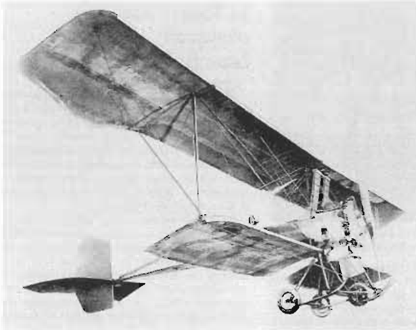
Breguet type III à moteur Canton-Unné sept cylindres en étoile fixe de 85 ch, tel qu'on peut le voir dans la chapelle du Musée des Arts & Metiers à Paris. (Cliché CNAM).
