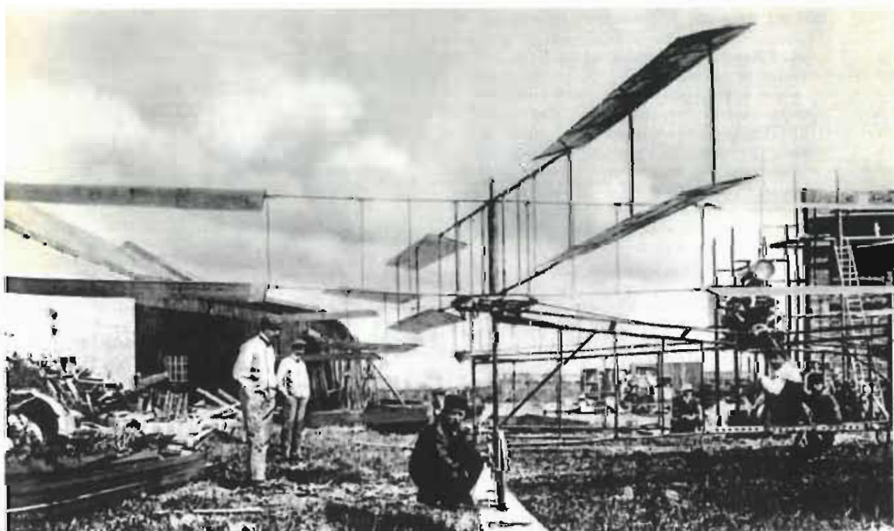
Le gyroplane Breguet-Richet n° 1, construit pendant l'hiver 1906-1907. On voit le moteur Antoinette à droite. Louis Breguet est debout à gauche. (Archives de l'Aéro-Club de France).
