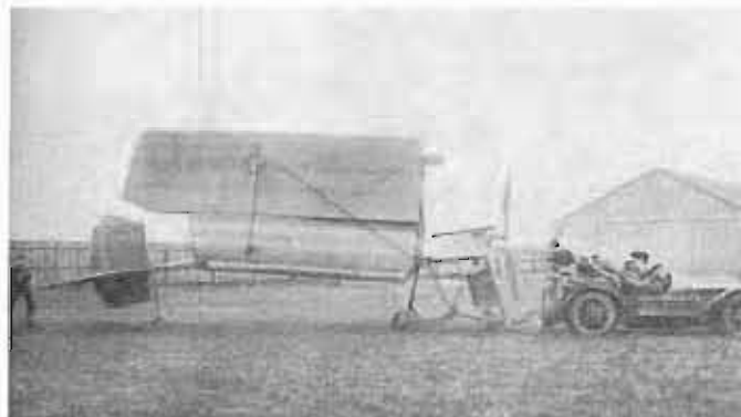
Breguet militaire type 1911-1912 à moteur Gnome prêt à être transporté. Les pales de l'hélice et les ailes se replient. (L'illustration).
